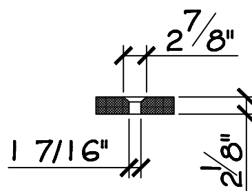
DÉTAIL DRAIN
