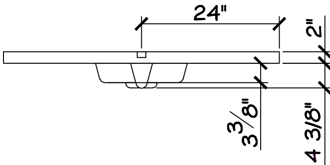
ÉLÉVATION
