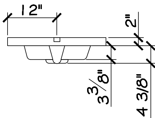
ÉLÉVATION
