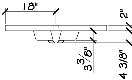
ÉLÉVATION
