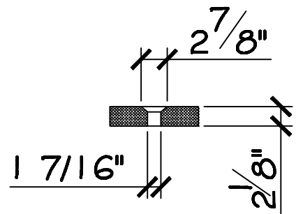
DÉTAIL DRAIN
