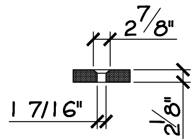
DÉTAIL DRAIN
