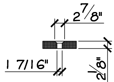
DÉTAIL DRAIN
