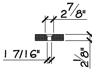
DÉTAIL DRAIN
