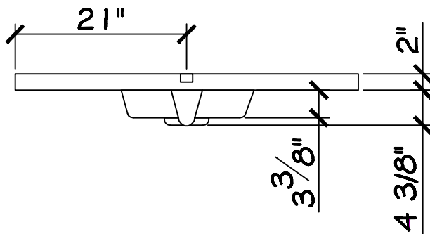
ÉLÉVATION
