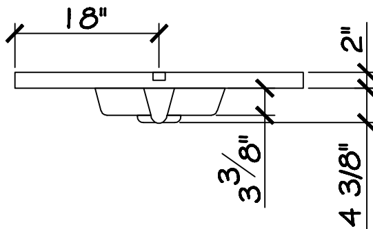
ÉLÉVATION
