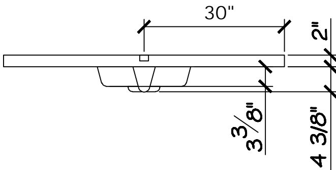
ÉLÉVATION
