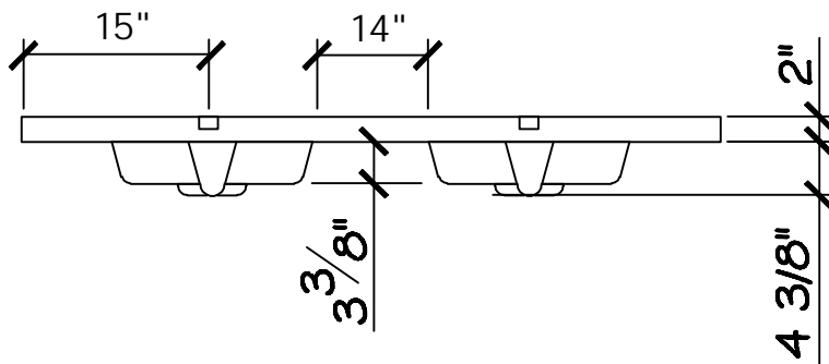
ÉLÉVATION
